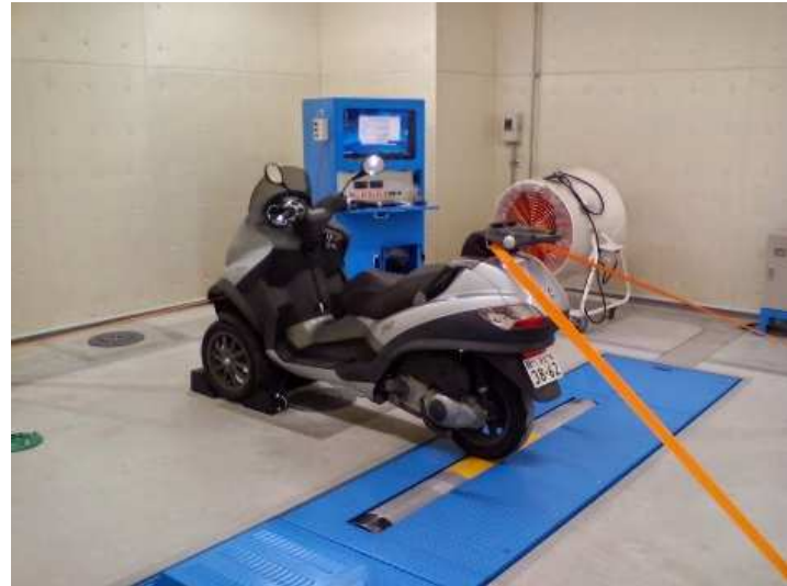
【駆動評価装置Ⅱ】
